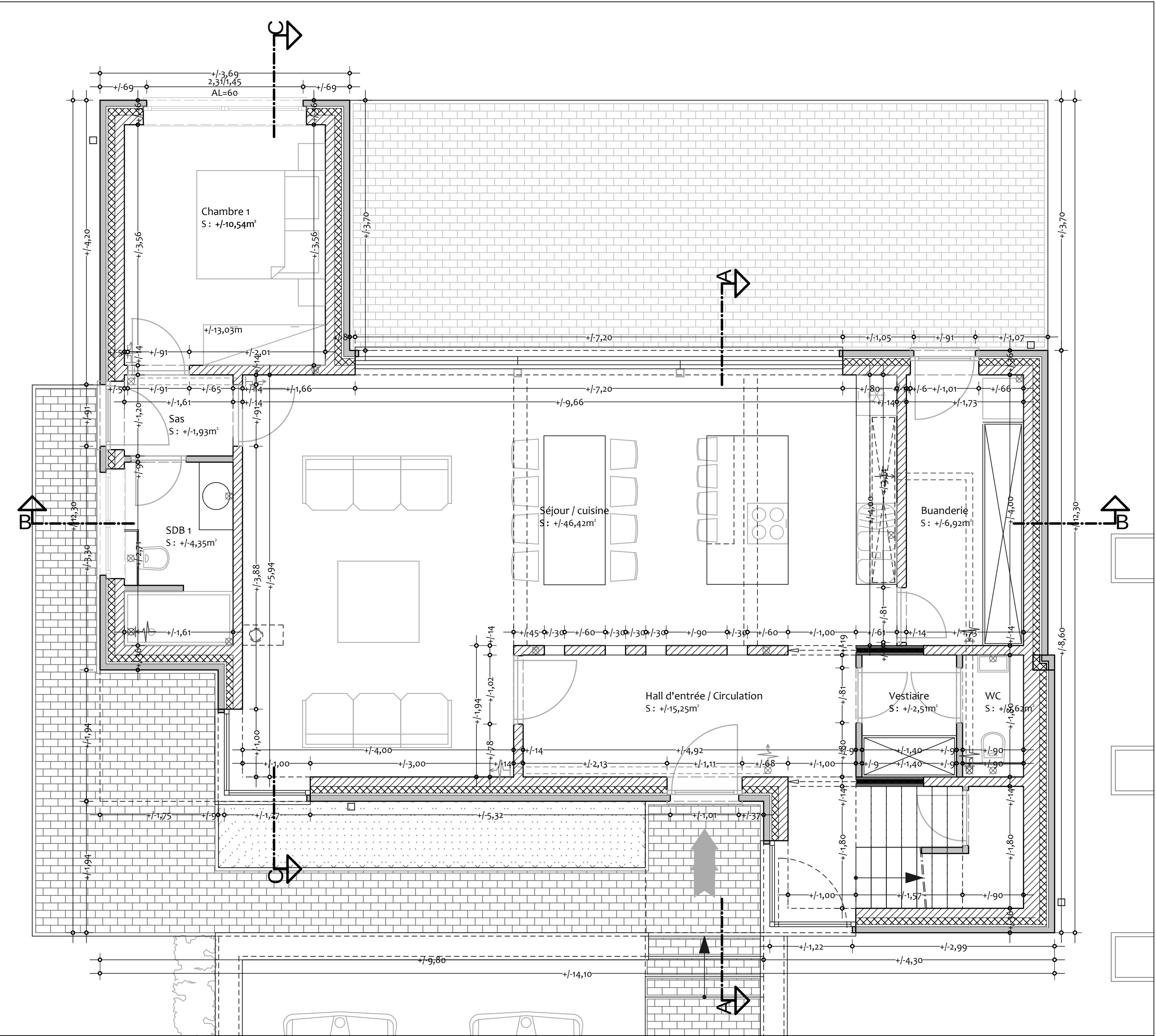
Vue en plan Rez-de-Chaussée
