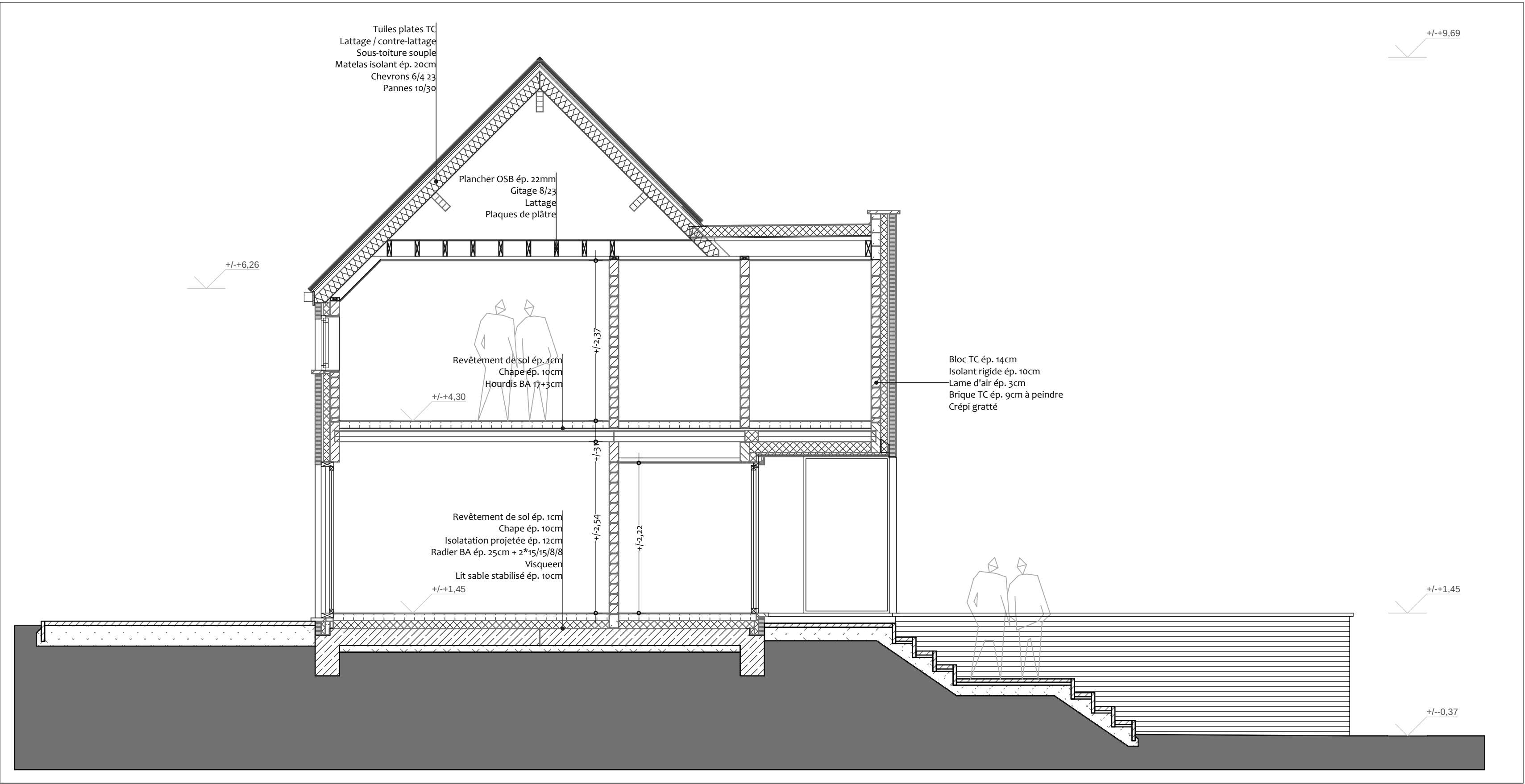
Coupe AA
